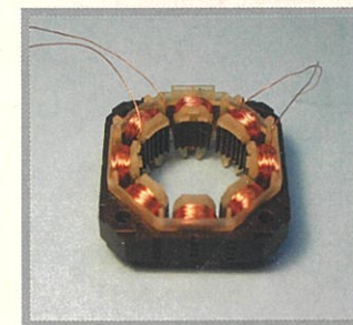
インナー巻
