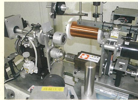
α巻線
