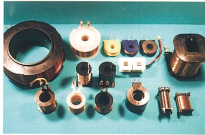
コイル各種
