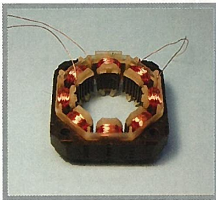
インナー巻
