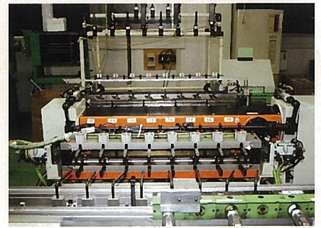
量産向 NC 巻線機 スピンドル
